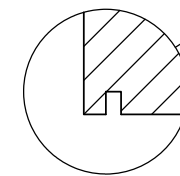
DETAIL F OPTIONAL DRIP GROOVE SCALE 1 : 1
